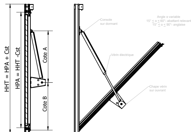
A-A ( 1:15 )
